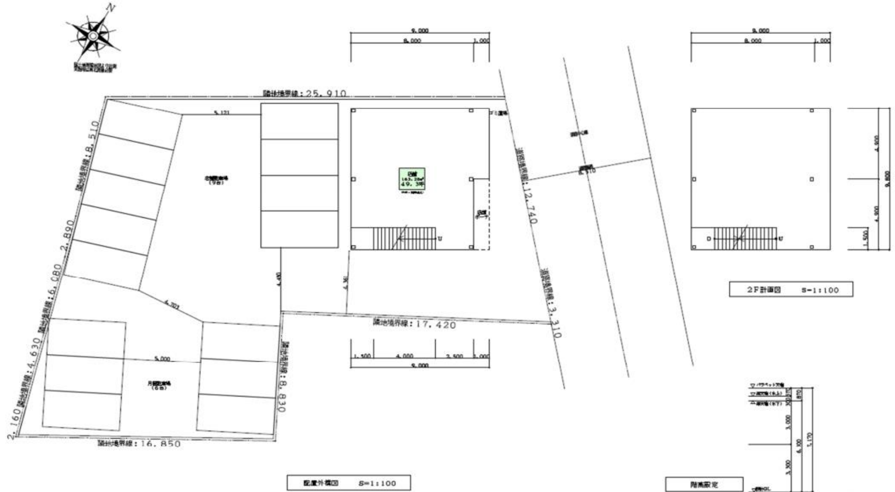
配置外構図
